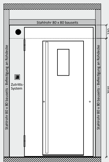
Ansicht Kundenseite
